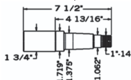
A-SP1750 Spindle
