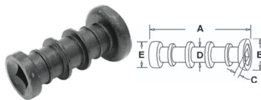
A-VLH6702 Rib Spool
