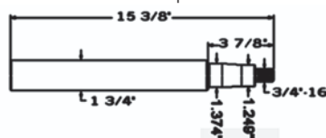
A-SP2500 Spindle
